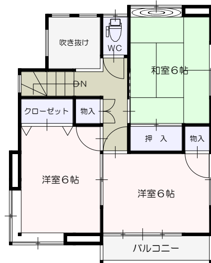
■2階間取図
